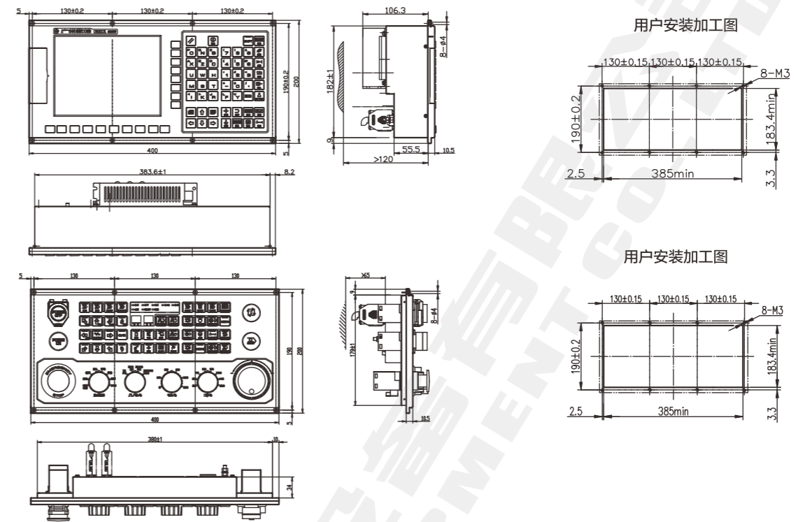
GSK 988TD (8.4 寸屏)外形安装尺寸 (横式)
