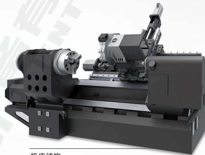
机床结构
