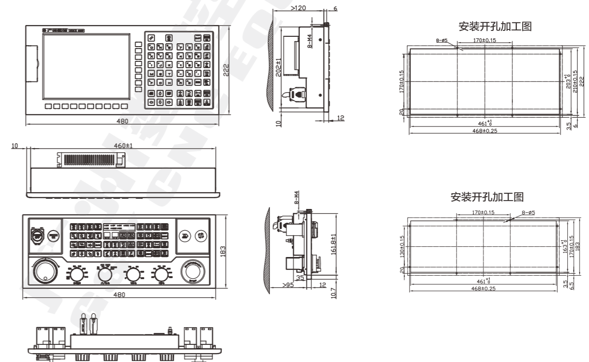
GSK 988TD (10.4 寸屏)外形安装尺寸 (横式)
