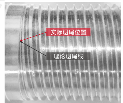
退尾终点清晰可见, 螺纹退尾长度小于1/3圈。
